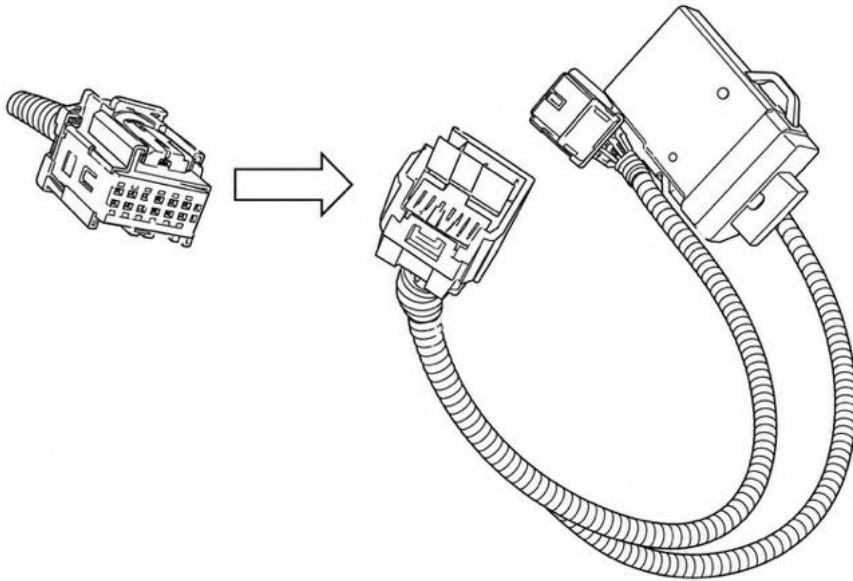
Conector original no encaixe do chicote E-Sync
