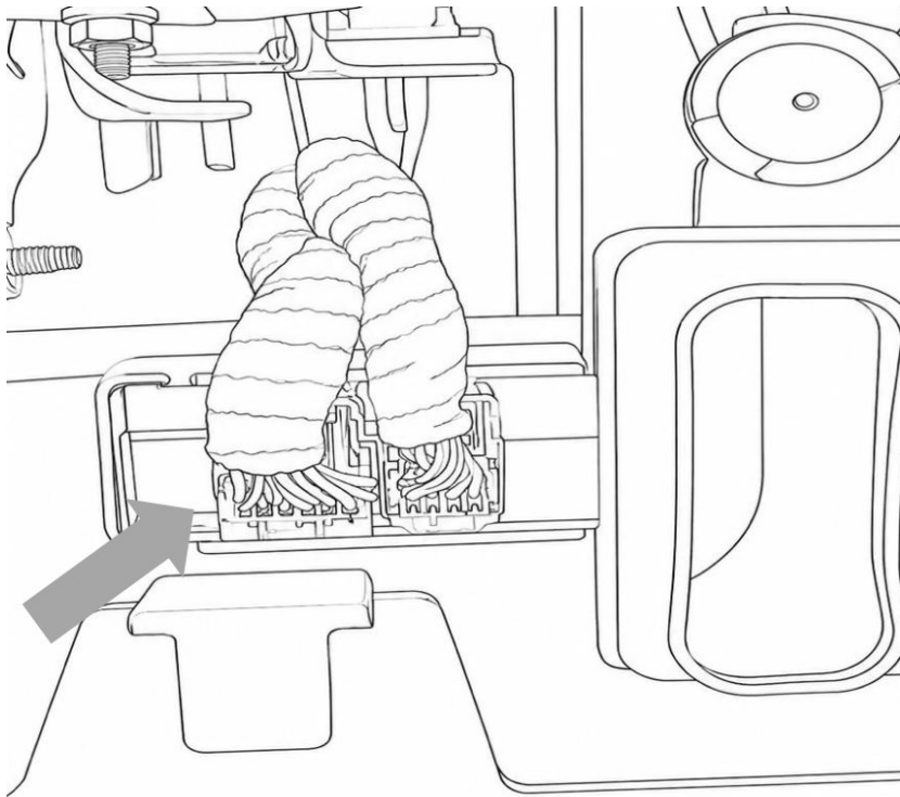
Vista inferior do porta-luvas
